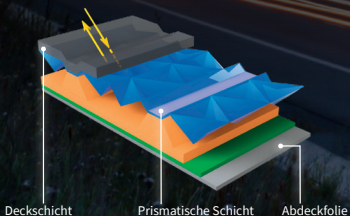
RA 2 C, RA 3 C - Aufbau mit Mikroprismen
