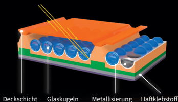
RA 2 B - Aufbau mit eingekapselten Mikroglasskugeln
