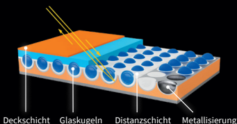
RA 1 A - Aufbau mit eingebundenen Mikroglasskugeln
